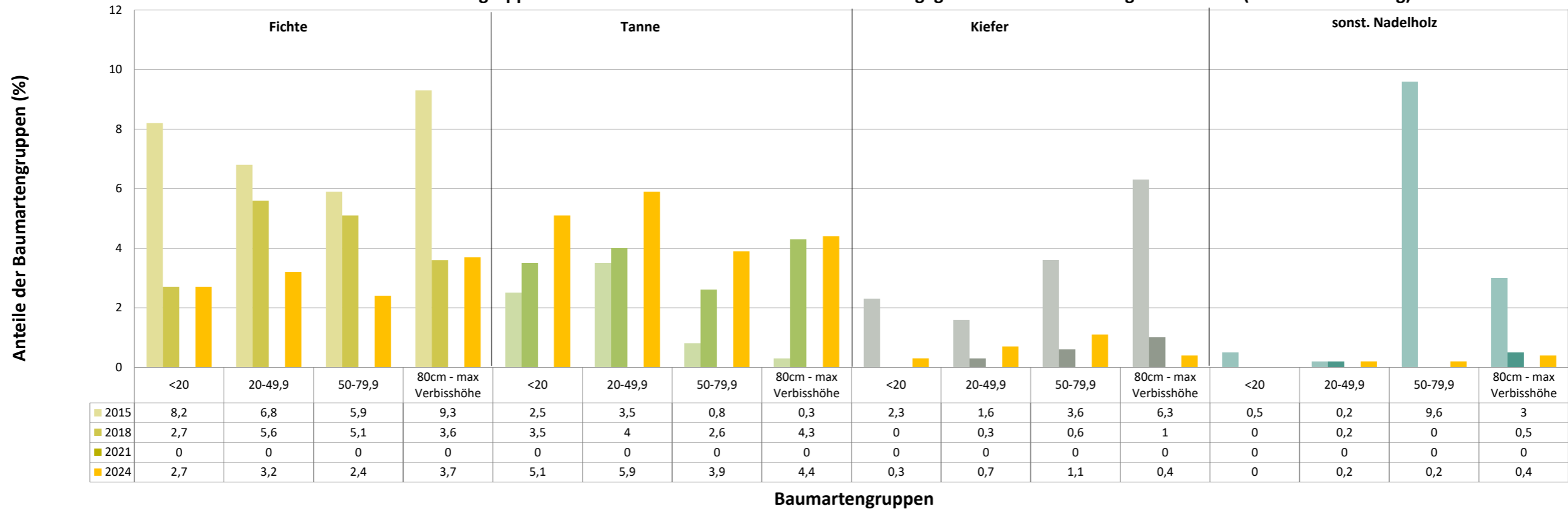
Anteile der Baumartengruppen in verschiedenen Höhenstufen für die die Hegegemeinschaft 414 - Steigerwald-West (Landkreis Bamberg)
