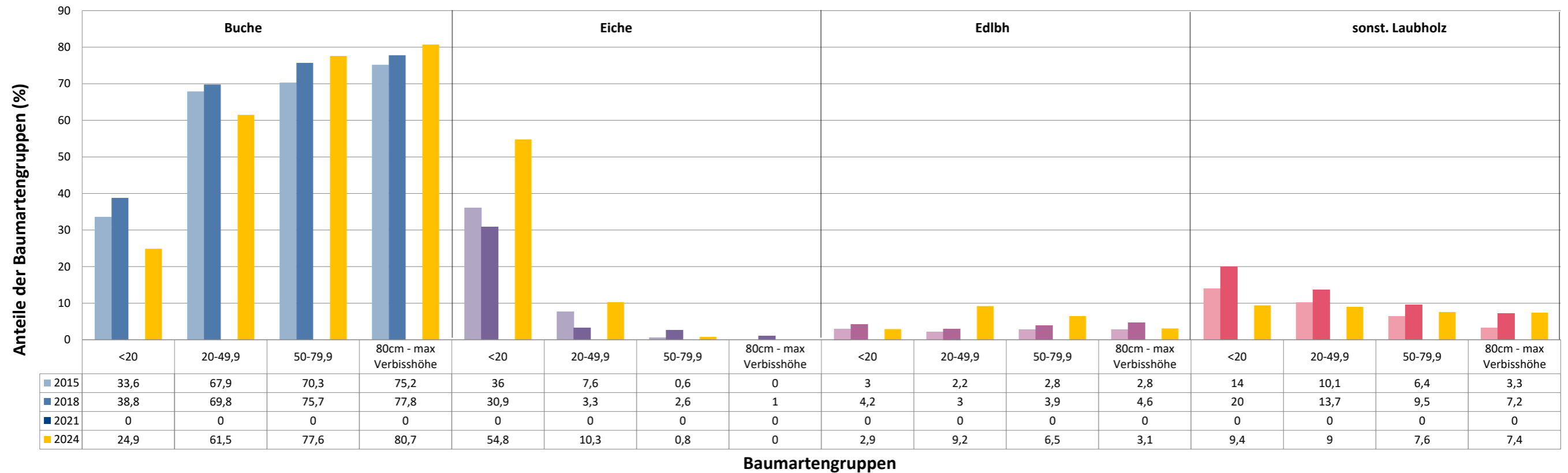
Anteile der Baumartengruppen in verschiedenen Höhenstufen für die die Heggemeinschaft 414 - Steigerwald-West (Landkreis Bamberg)
